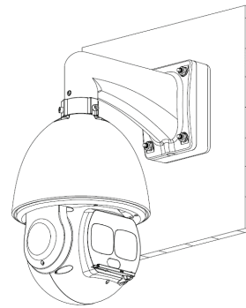
Installation mit PTZ Wandhalterung
