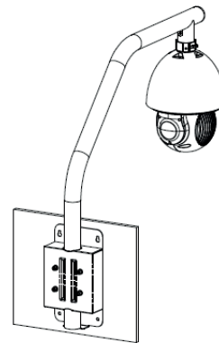
Installation mit Adapter NH-AD1
