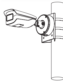
Installation mit runder Anschlussbox
